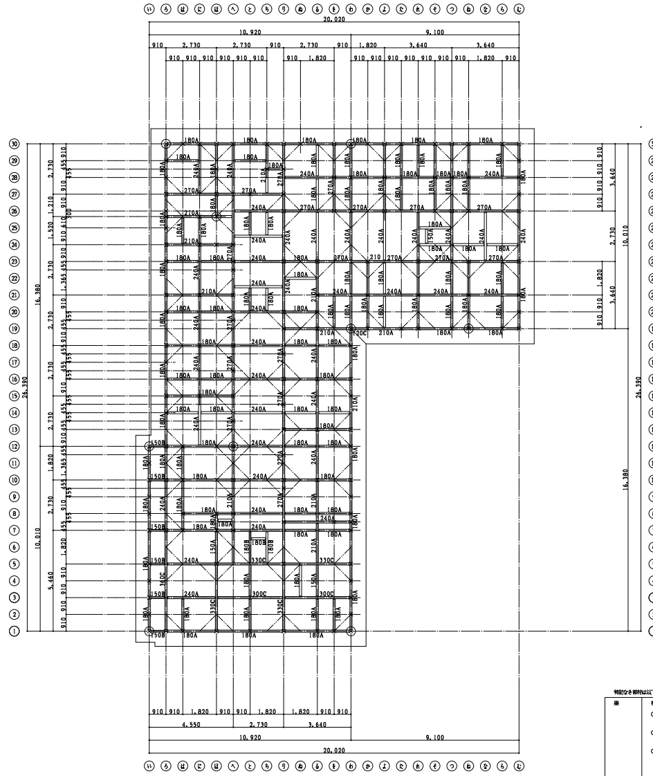
R階梁伏図 S:1/100 原縮率:縦縮率1/2m N50150以下引付5+火打5.2.5#以下
